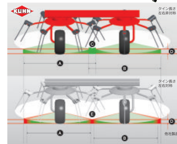
A 左ローターの作業幅 B 右ローターの作業幅 C 重複箇所 D 作業高 E 要注意箇所
