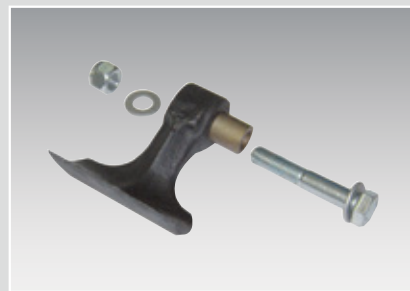
特許所有の06ハンマーナイフは熱処理加工を施したナイフと特殊なブッシングにより装着
