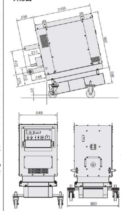
オートヒッチ対応型 日農工標準OS (O・I型兼用) TSN-8S
