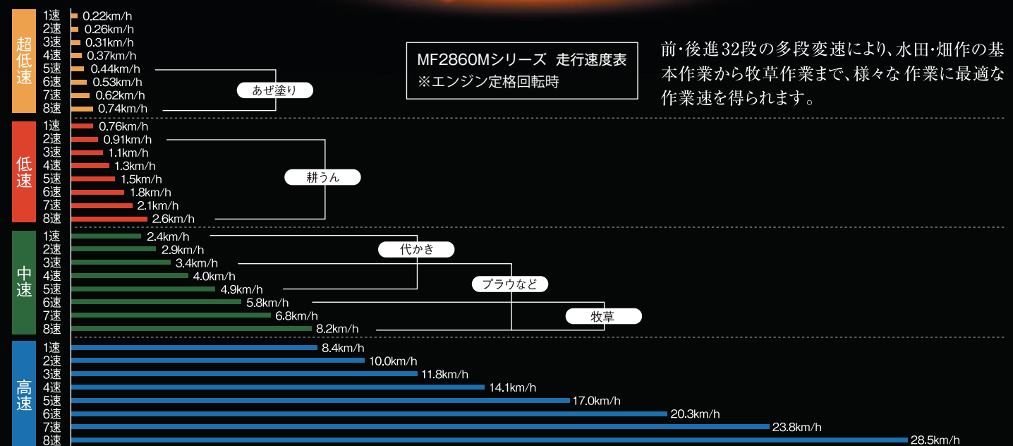
車速グラフ
