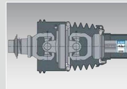
広角 PTO シャフト
